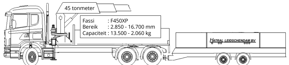
3-Assige Aanhanger. Laadvermogen: 7000 mm. Laadvermogen 13.870 kg
